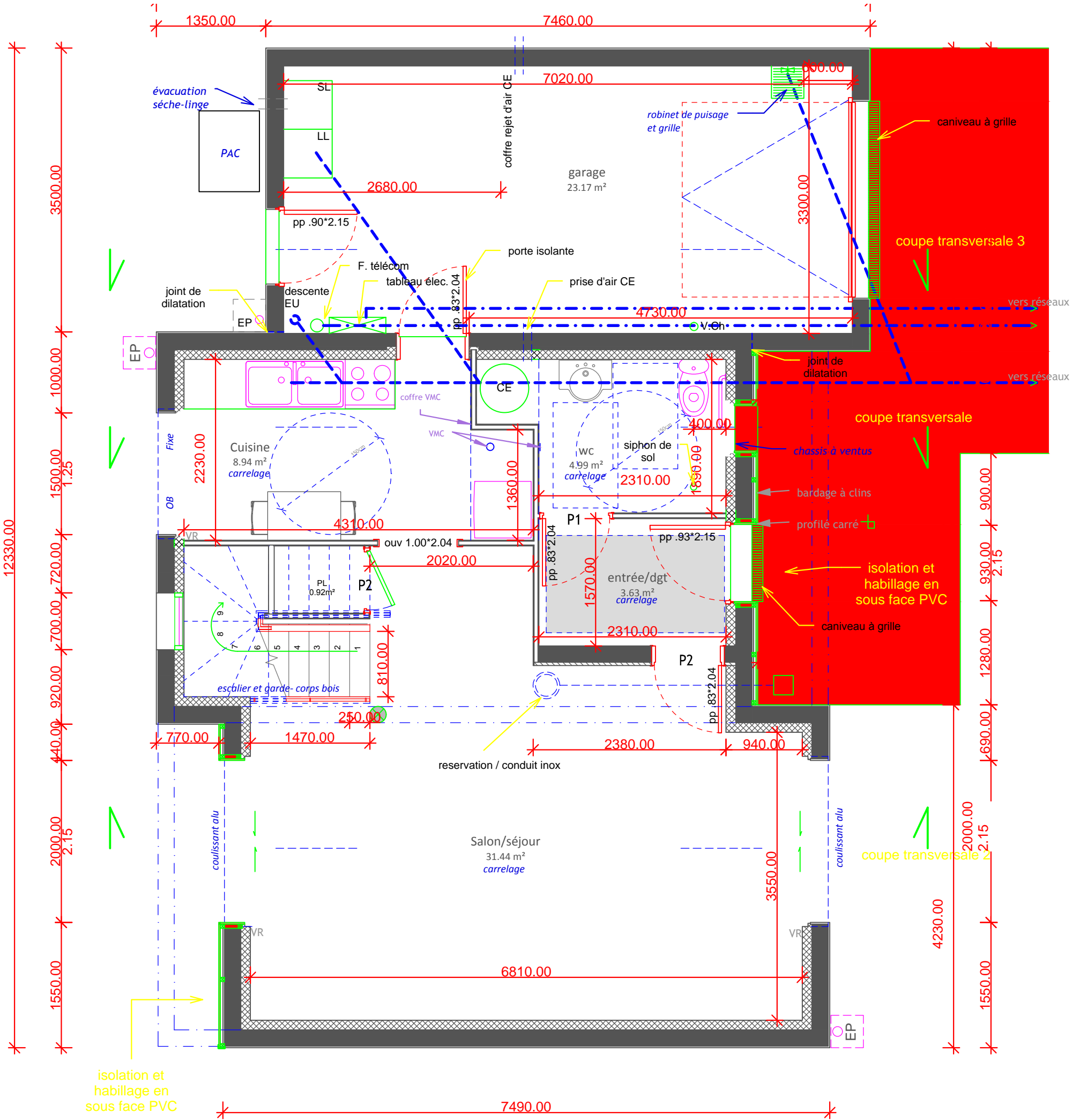
Type2 4P Niveau 0 1 : 50
