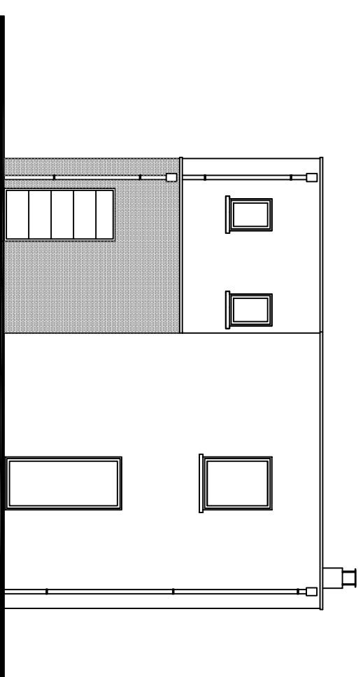
ÉLÉVATION NORD
