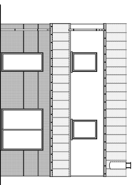
ÉLÉVATION SUD
