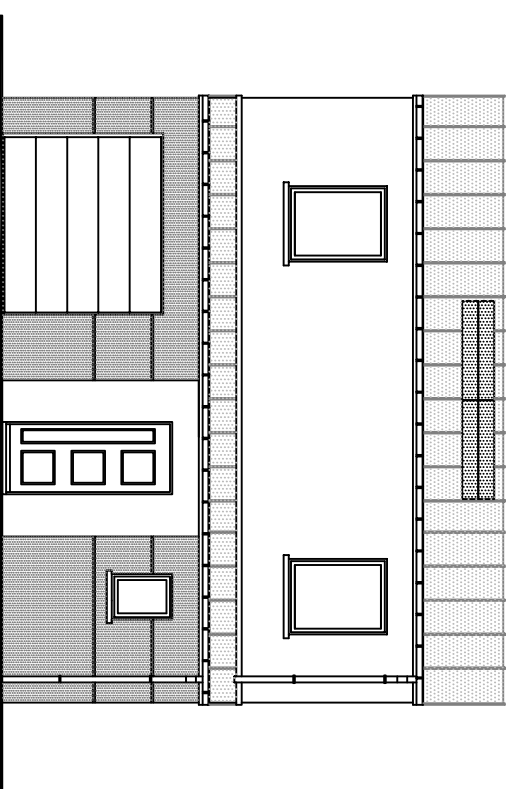
ÉLÉVATION NORD
