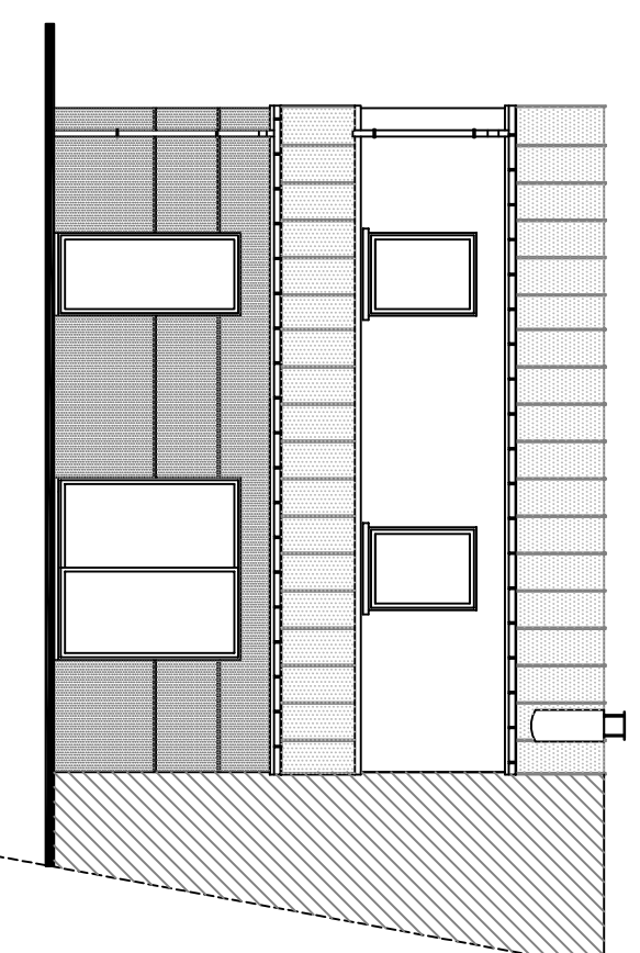
ÉLÉVATION SUD
