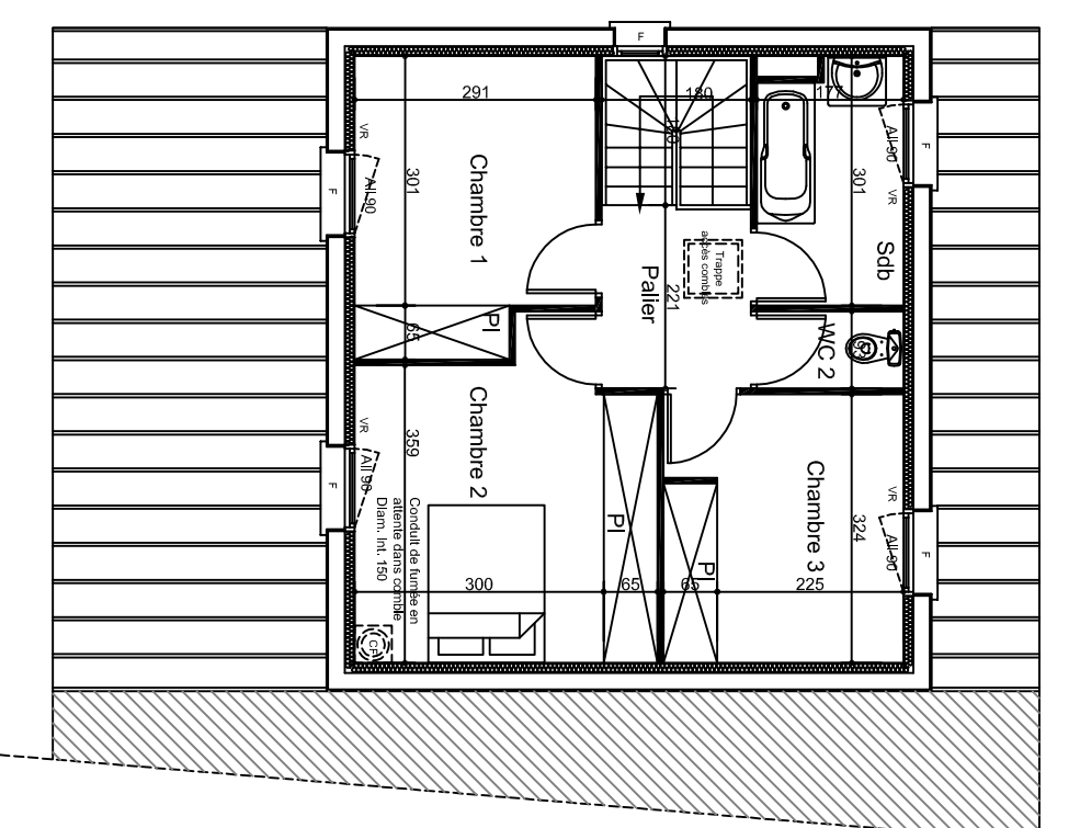
ÉTAGE
